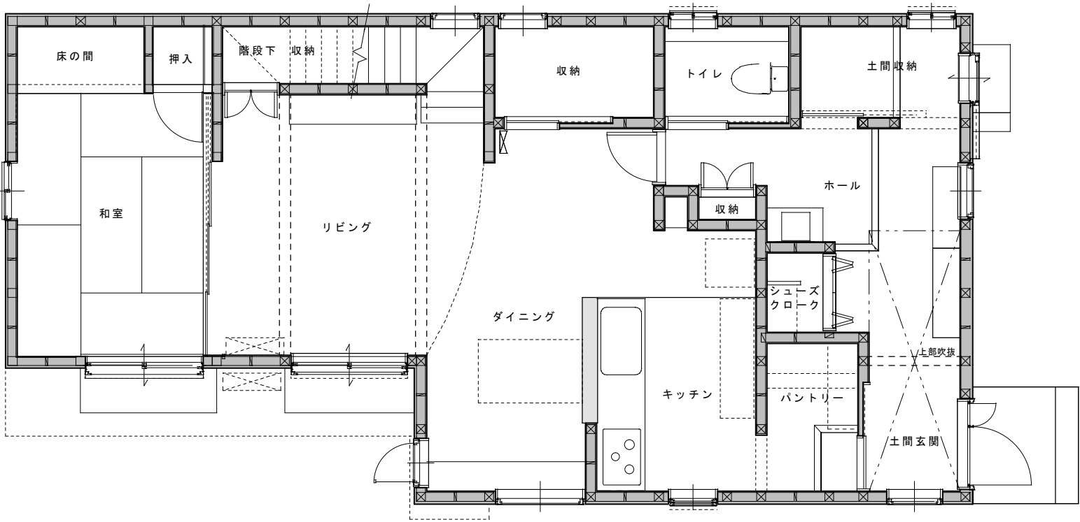
1 階 平 面 図
